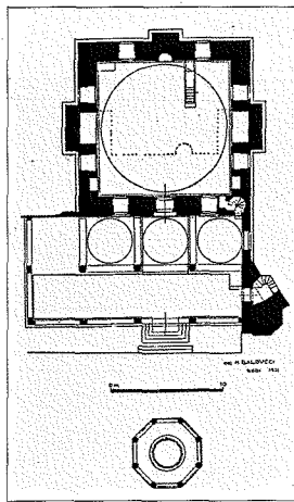
İbrâhîm Paşa Camii'nin planı
